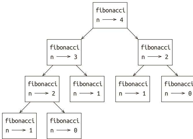
Рис. 11.2. Граф вызова
